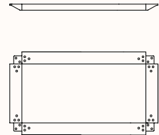
Frame U84 OW 800mm OD 450mm OH 40mm
